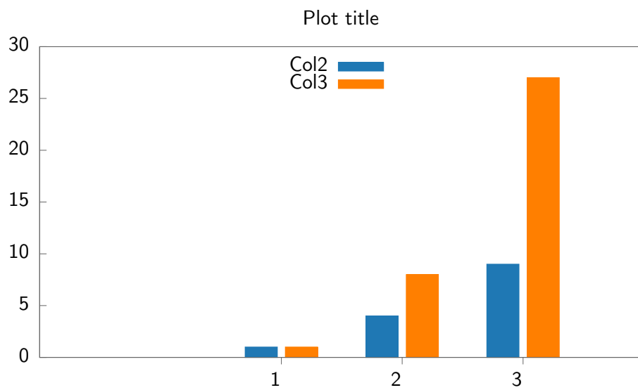
Figure 1: График параболы
